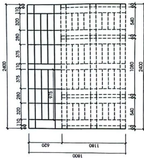
CHI TIẾT HOA SẮT CỦA S1 CẢI TẠO (SL: 05 BỘ)
